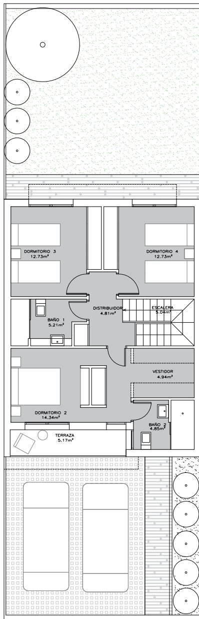
PLANTA PRIMERA
