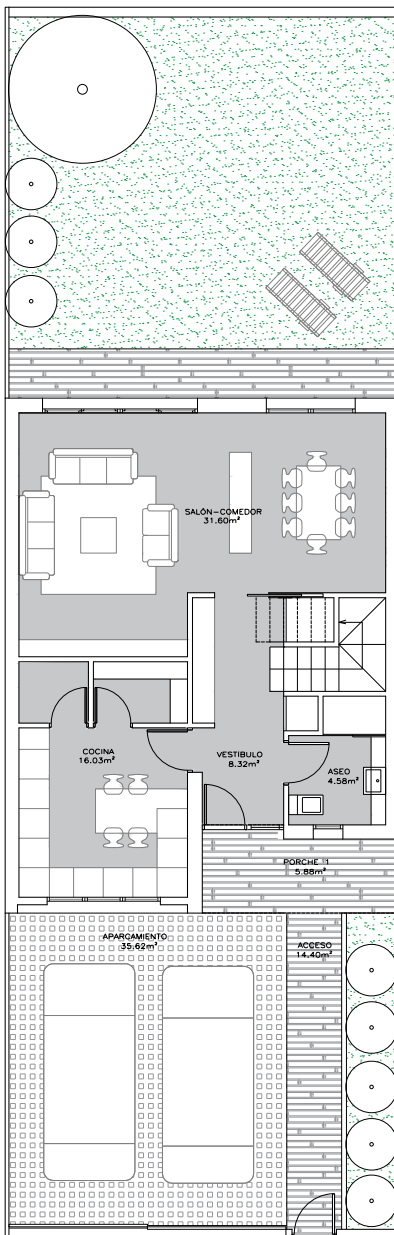
PLANTA BAJA
