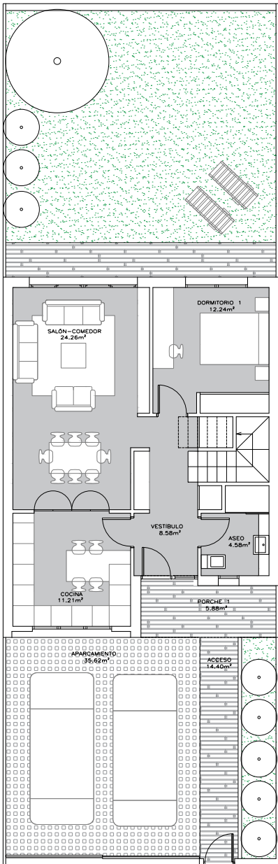
PLANTA BAJA
